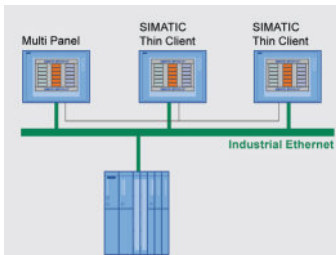
Thin Client'tan Sm@rtServer Operatör Paneline bağlantı
