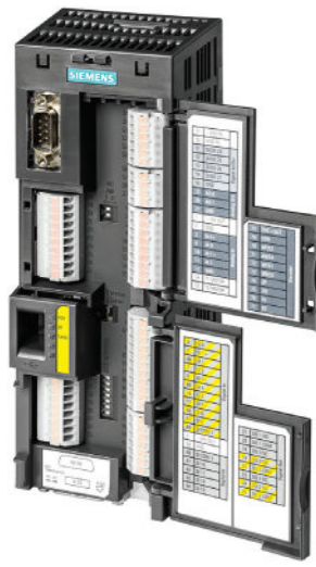
SINAMICS G120 Kontrol Üniteleri
