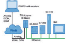
Teleservis Adaptörü
